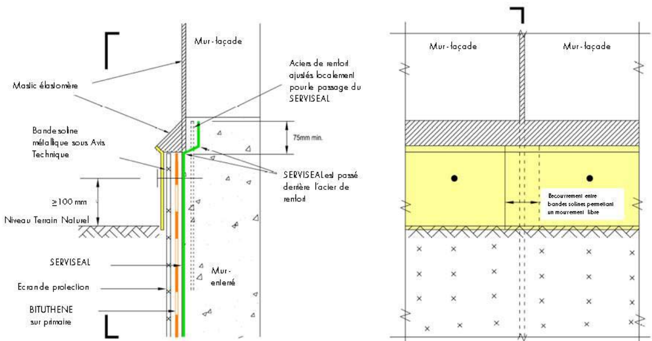
Figure 9 : Arrêt en partie haute au droit d'un joint de dilatation
