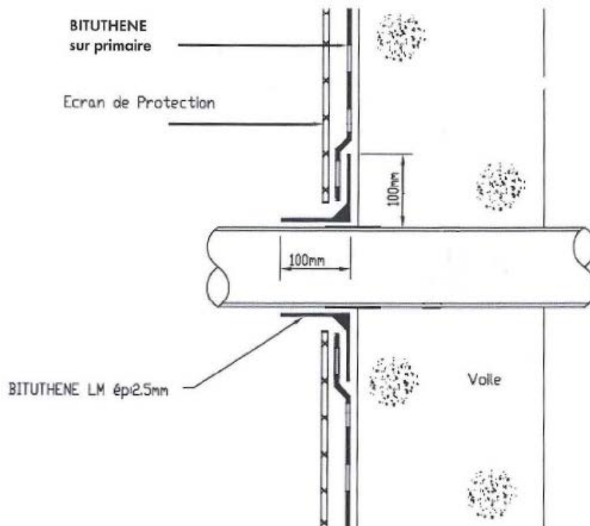
Figure 10 : Traitement des traversées
