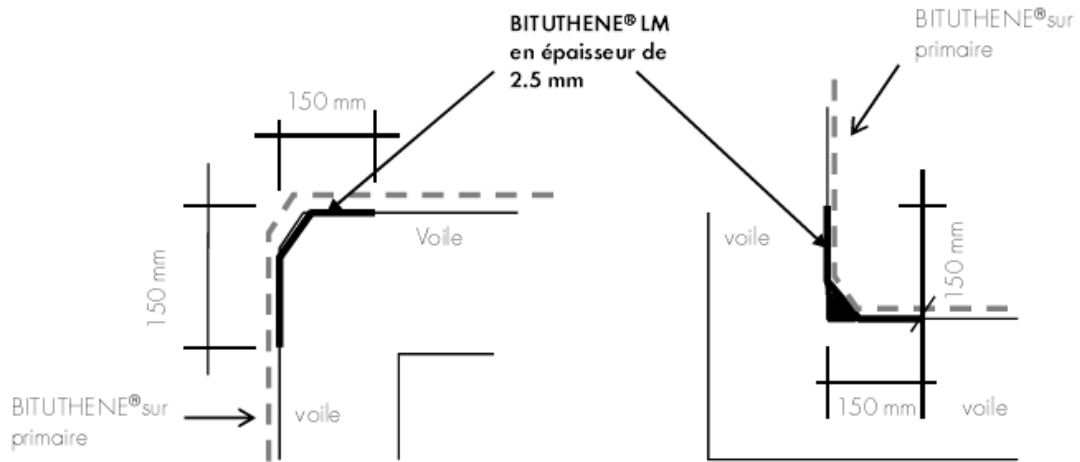
Figure 6 : Traitement des angles par le mastic BITUTHENE LM
