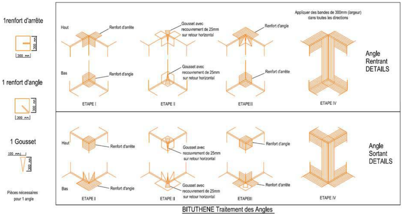
Figure 3 : Principe de traitement des différents angles préalablement au renforcement par la bande adhésive PERMA BARRIER ou par doublement de la membrane BITUTHENE
