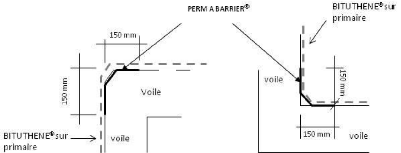
Figure 4 : Traitement des angles rentrants et sortants aux jonctions voile-voile par renfort à l'aide de la bande adhésive PERMA BARRIER
